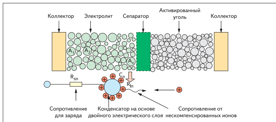
Рис. 4. Схематическое изображение многослойной структуры активированный уголь/электролит
