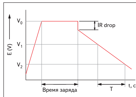
Рис. 8. Зависимость напряжения для ионистора от времени
