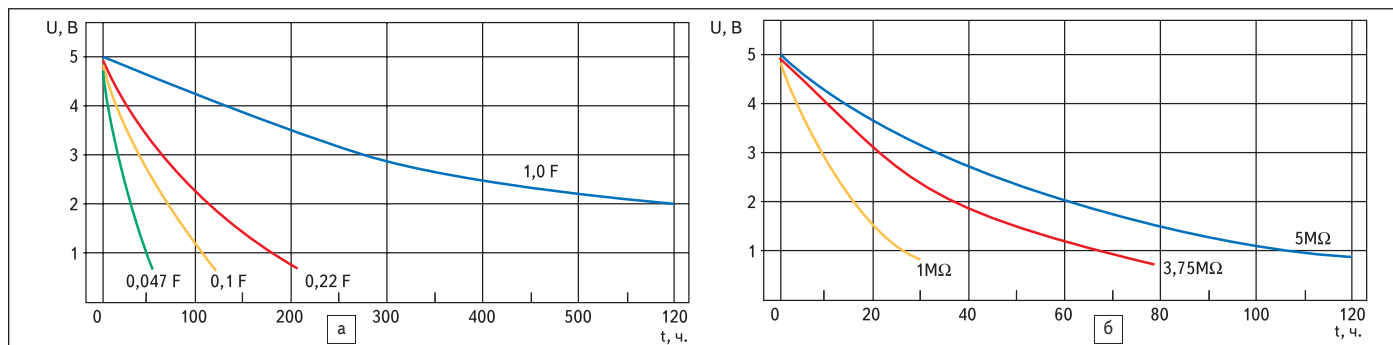
Рис. 14. Характеристика разряда для ионисторов различной емкости при сопротивлении 1 МОм (а) и в зависимости от сопротивления для EEC50HD473V (5,5 В, 0,047 Ф) (б). Условия заряда: 5 В, 24 часа, +20 °С
