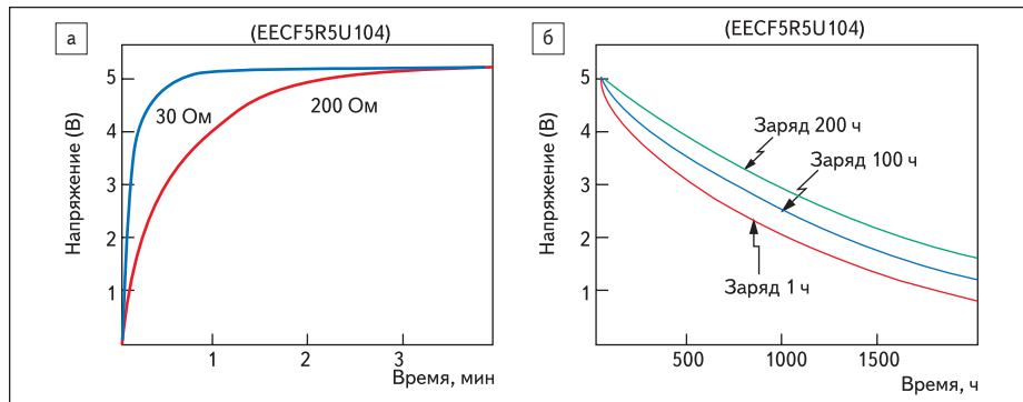
Рис. 9. Зависимость напряжения ионистора от времени заряда при различном сопротивлении (а) и времени разряда при различном времени заряда (б)
