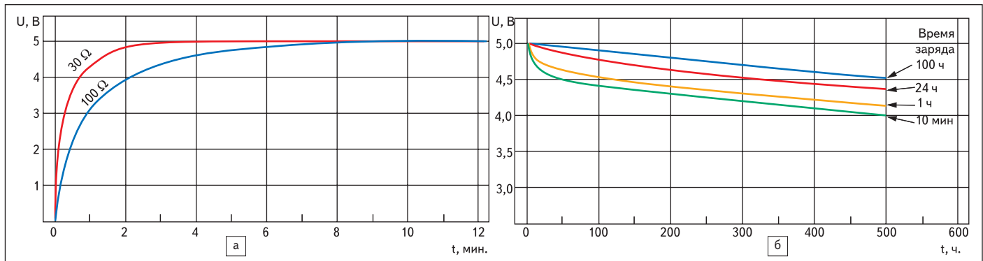
Рис. 12. Характеристика заряда (а) и саморазряда (б) для EECF5R5U105 (5,5 В, 1,0 Ф) при +20 °С
