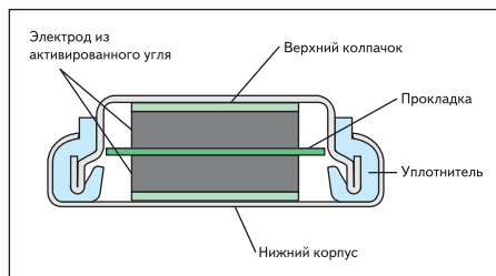
Рис. 3. Одна из возможных конструкций ионистора в поперечном разрезе на примере EN серии Panasonic
