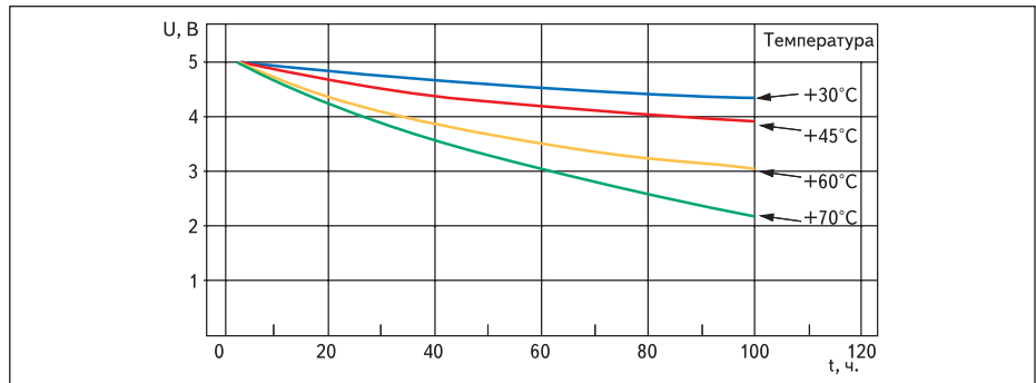
Рис. 13. Характеристика саморазряда в зависимости от температуры для EEC50HD104V (5,5 В, 0,1 Ф) Условия заряда: 5 В, 24 часа
