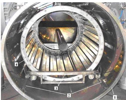
Рис.8. Внутренние элементы камеры установки VATT1600-4ДК
